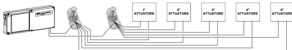
Fig. 5: Esempio di collegamento di un massimo di 5 attuatori per canale tramite morsetti a cappuccio.
