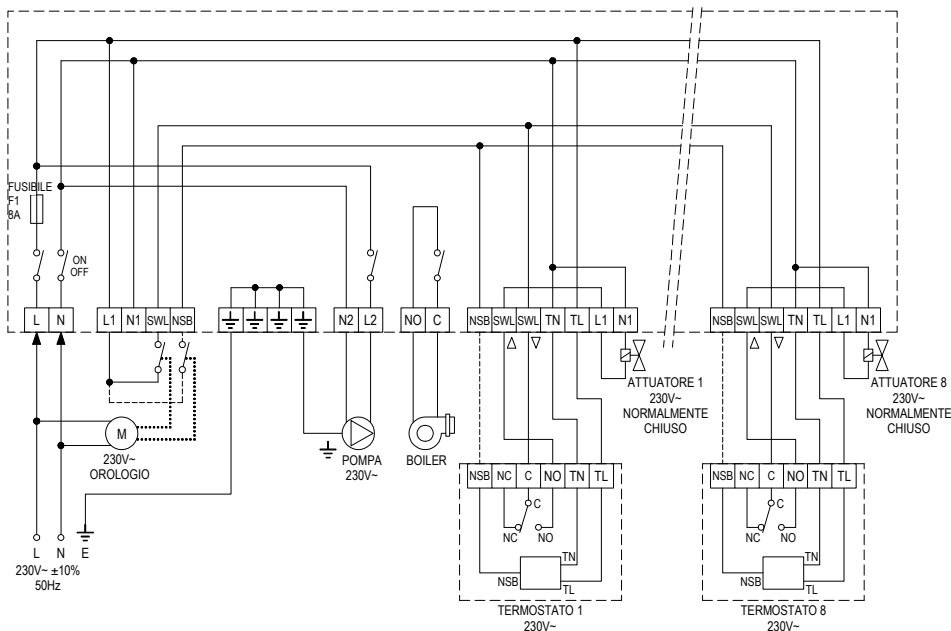
Fig. 4: Schema di collegamento.
